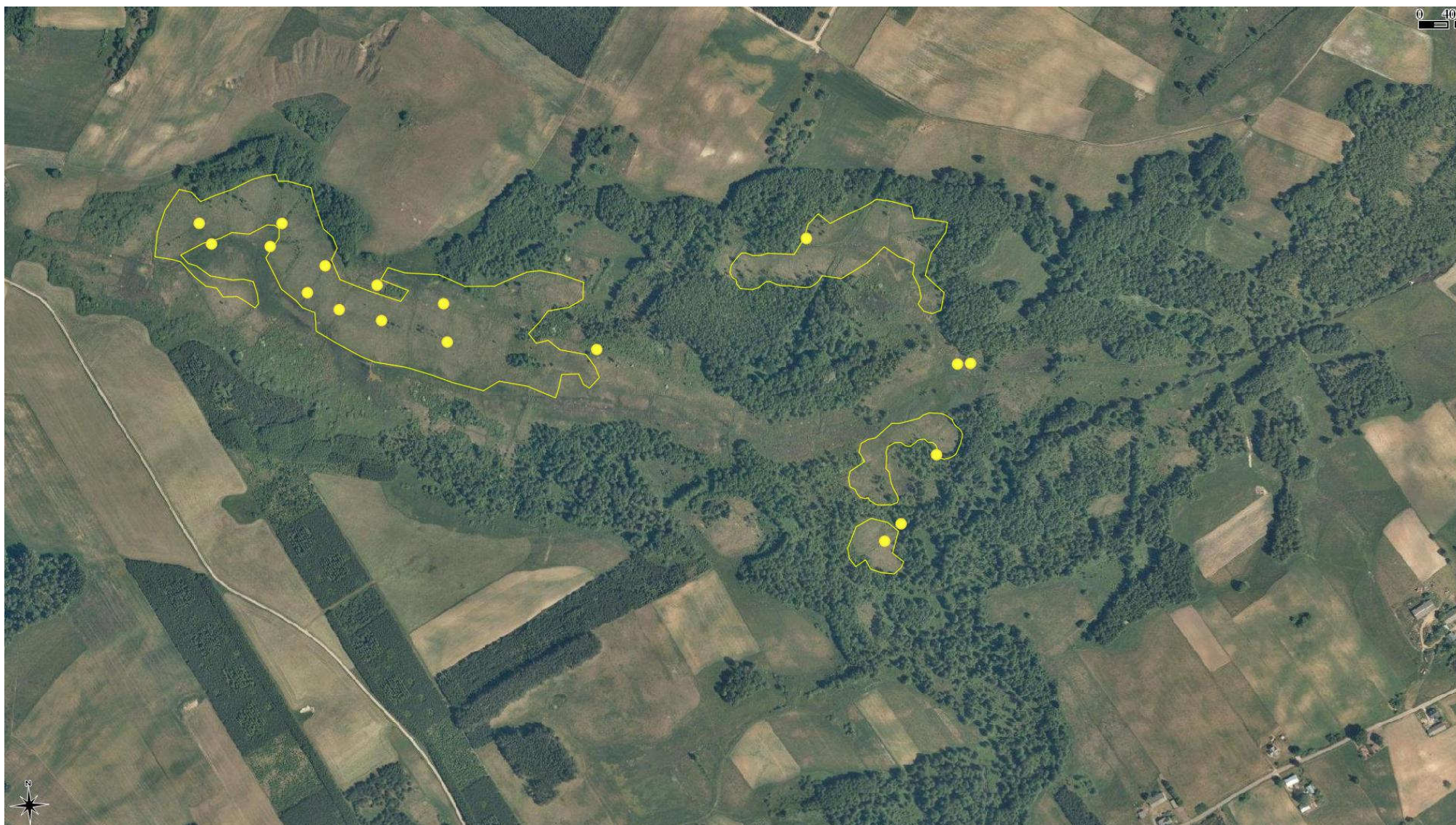
Lokalizacja zabudowy biologicznej na obiekcie Rudawki, gmina Rutka Tartak, powiat suwalski, woj. podlaskie
